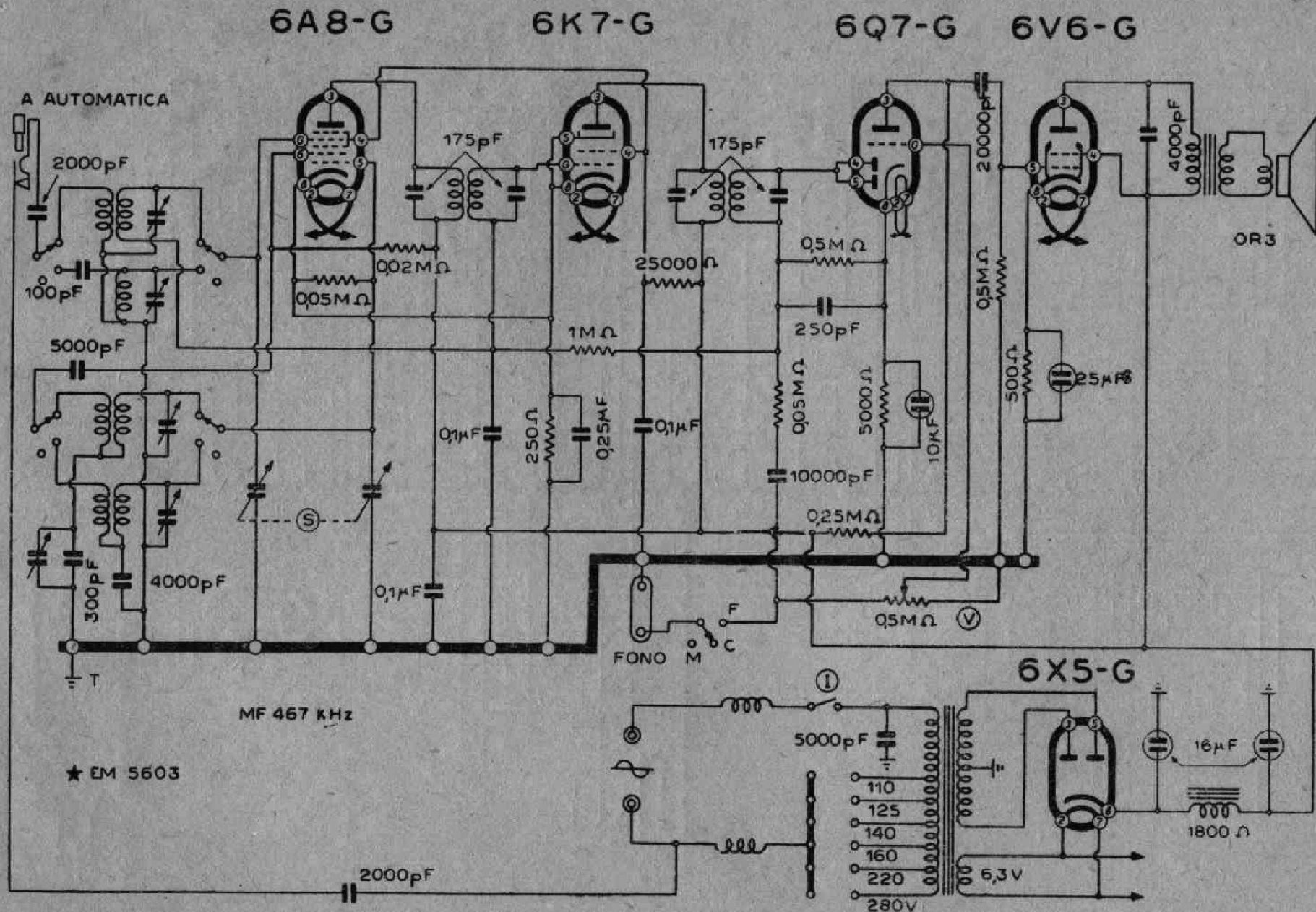
Lo schema elettrico del mod. 522
